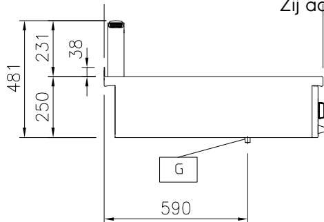
Zij aanzicht
