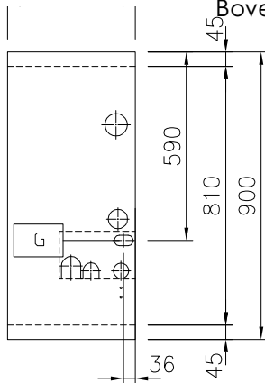
Boven aanzicht
